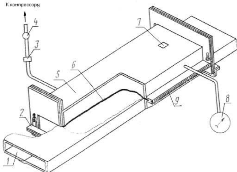
1 - образец; 2 - опоры; 3 - трехходовой кран; 4 - вентиль; 5 - короб; 6 - резиновая мембрана; 7 - предохранительный клапан; 8 - манометр; 9 - крепежные уголки
